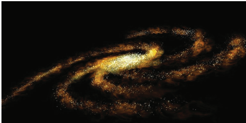
Gambar 6.3 Galaksi Bima Sakti Sumber: kompas.com/nasa (2020)
